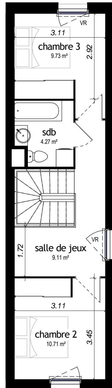
1er Etage
